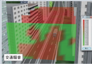
▲コンタ図(左)、コンタライン(右)の表示に対応
