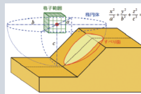
▲すべり面自動探索機能のイメージ図
