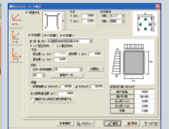
▲剛比によるモーメント分配入力画面
