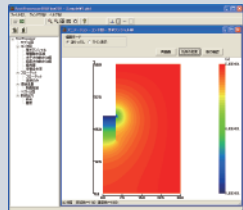
▲PostProcessor等ポテンシャルコンタ図
