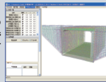
▲3D配筋機能
