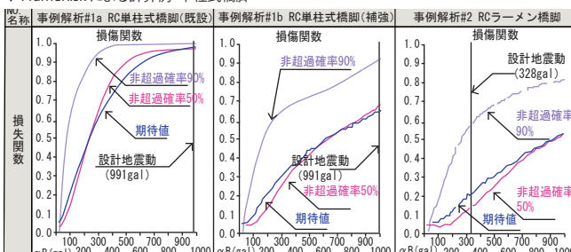
▼FrameRiskによる計算例:単柱式橋脚
