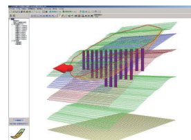
▼3D表示例 (DEM型3D: 杭配置図)
