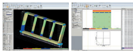
▲変形とコンクリートの損傷
