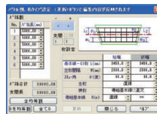
▼横断面設定
