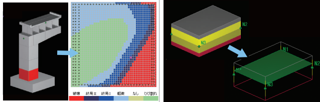
▼ファイバー要素の結果画面(右:断面)
