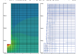
▼最終掘削時の変形と変位コンタ図
