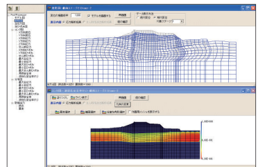
▼河川堤防地震時自重変形解析図(変形図、FL図)
