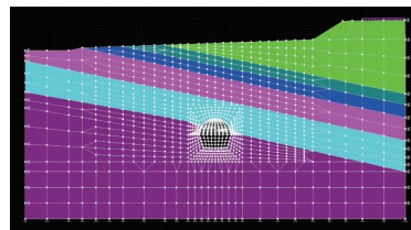
▼トンネル掘削解析-プリプロセス
