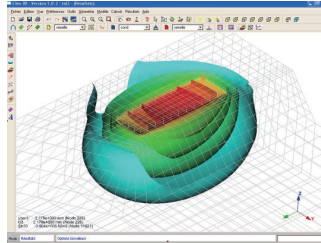
▼堤防に近い浅基礎(変位ノルムの等値曲面)
