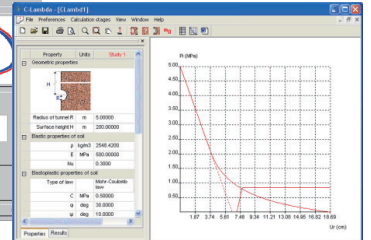
▼収束拘束曲線の決定
