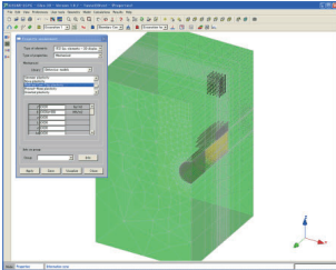
▼3Dトンネルモデルプロパティ設定
