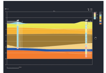
▼断面図のDXFファイル出力
