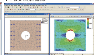
▼平板要素解析結果
