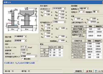
▼初期設定画面
