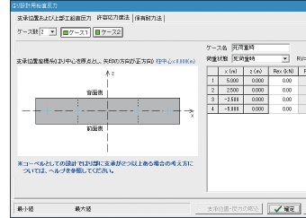
▼はり主鉄筋入力
