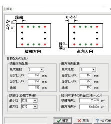
▼配筋条件の設定
