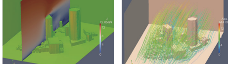
▲中目黒駅周辺のメッシュと風速分布図(コンター/ベクトル)
