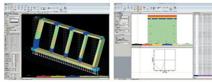
▲変形とコンクリートの損傷 ▲断面内の損傷状況および応力ひずみ履歴
