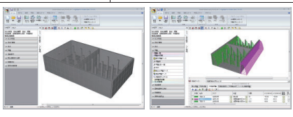
▲変形とコンクリートの損傷 ▲断面内の損傷状況および応力ひずみ履歴
