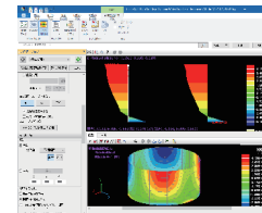
▼3次元コンタ図と2次元切断面図
