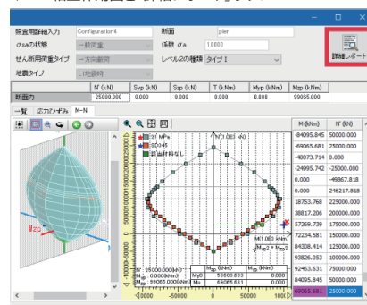
▼M-N相互作用図と「詳細レポート」ボタン
