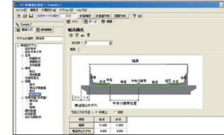
▼横桁の設計、横方向の設計 断面形状
