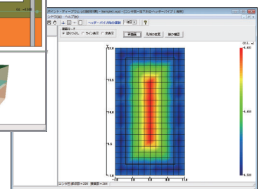
▼等水線図
