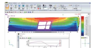
▼地盤と構造物の一体解析結果
