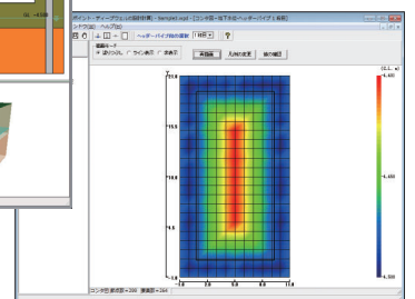
▼等水線図
