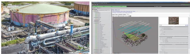
▲iTwin Capture Modeler: リアリティメッシュ(写真テキストチャ付3Dモデル)により、現実のコンテキストを正確に反映(左)/写真から空中三角測量を自動実行可能(右)
