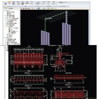
▲橋台堅壁配筋図
